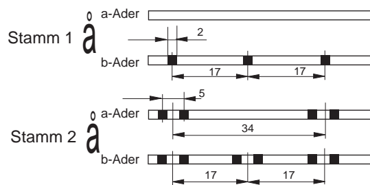
Ringkennzeichnung (Maße in mm)
